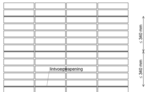
Aanzicht van in tegelverband uitgevoerd metselwerk voorzien van lintvoegwapening
